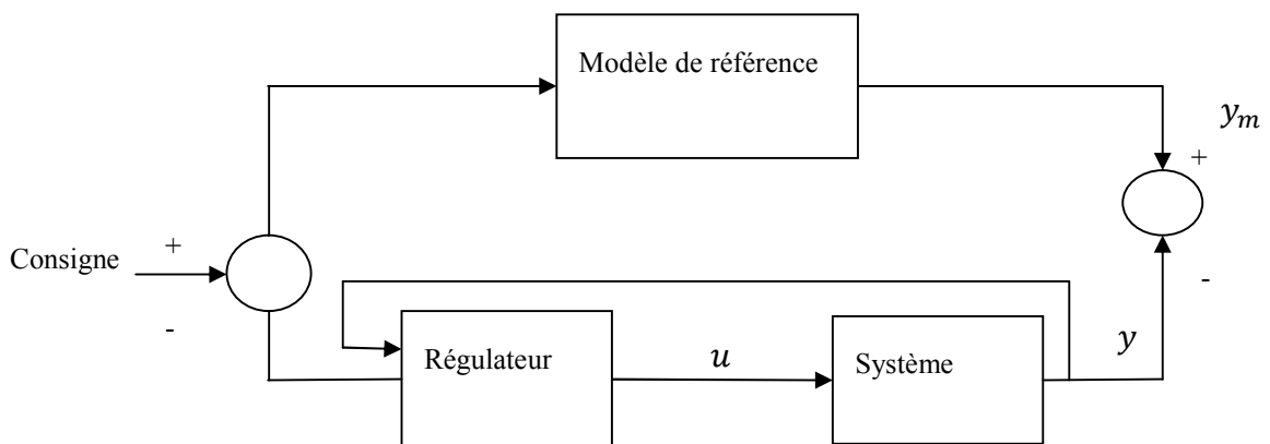
Figure II.6 : Commande adaptative à modèle de référence.
