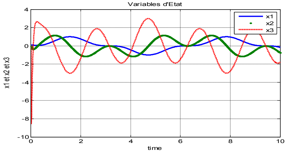
Figure III.2 : Signaux des variables d'état.
